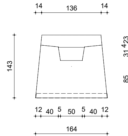
Vooraanzicht
